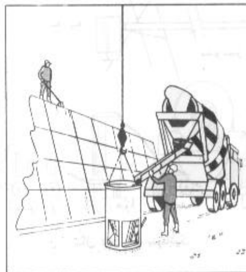
شکل ۴۴. بتن ریزی به کک جام و حرنقبیل
