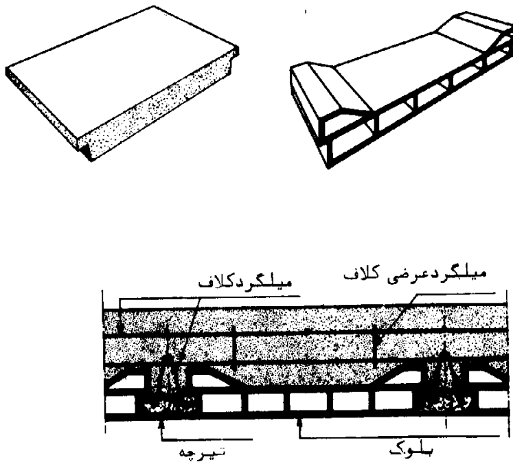
شکل ۲۳. استفاده از بلوکهای کم ارتفاع برای حذف قالب‌بندی کلاف بتنی
