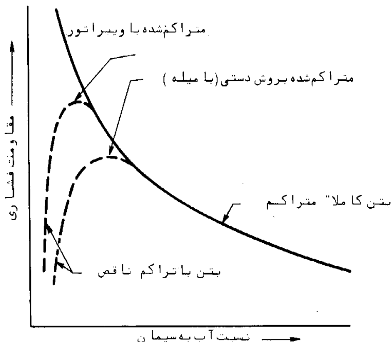
نمودار ۱. چگونگی تغییر مقاومت فشاری بتن برحسب تغییرات نسبت آب به سیمان آن
