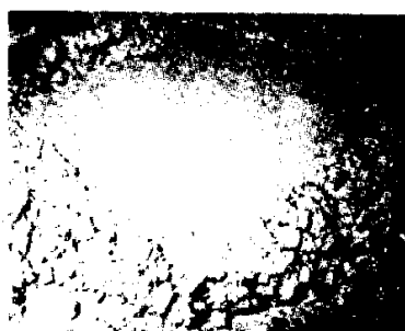
شکل ۹۸. سطح بتن مالکشی شده
