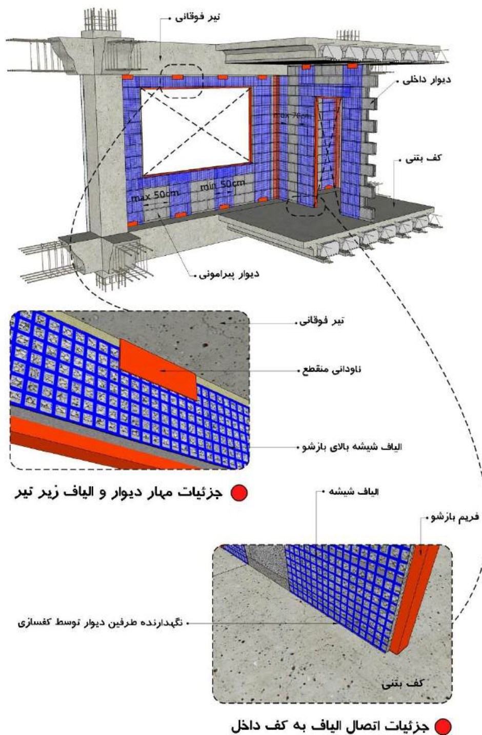
شکل ۳-۵- تسلیح دیوار در مجاورت بازشو با استفاده مش الیاف - وجه داخلی دیوار
